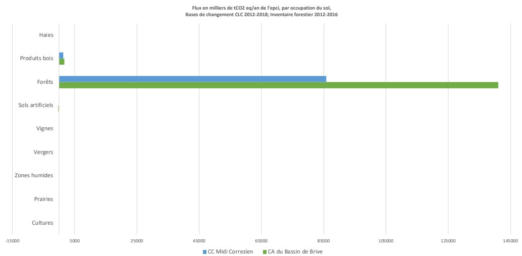
Flux de carbone sur le territoire (source outils ALDO, Traitement EAU)
